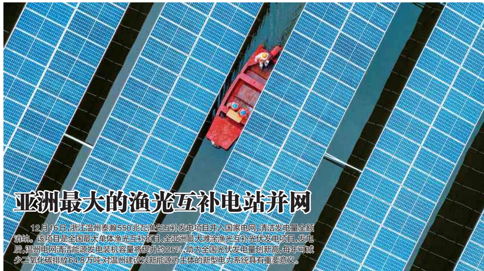
12月16日, 浙江温州泰顺550兆瓦渔光互补光伏发电项目并入国家电网, 清洁能源全面并网发电。该项目是全国最大单体渔光互补项目, 全面覆盖太湖流域渔业与光伏发电产业, 总装机100兆瓦, 年发电量1.5亿千瓦时, 减排二氧化碳约3.6万吨, 对推动浙江省新能源高质量发展具有重要意义。
